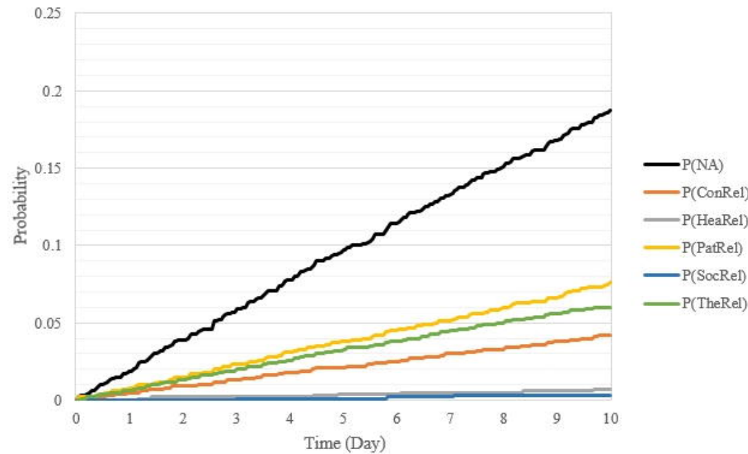
P(NA) and P(NAFs)
