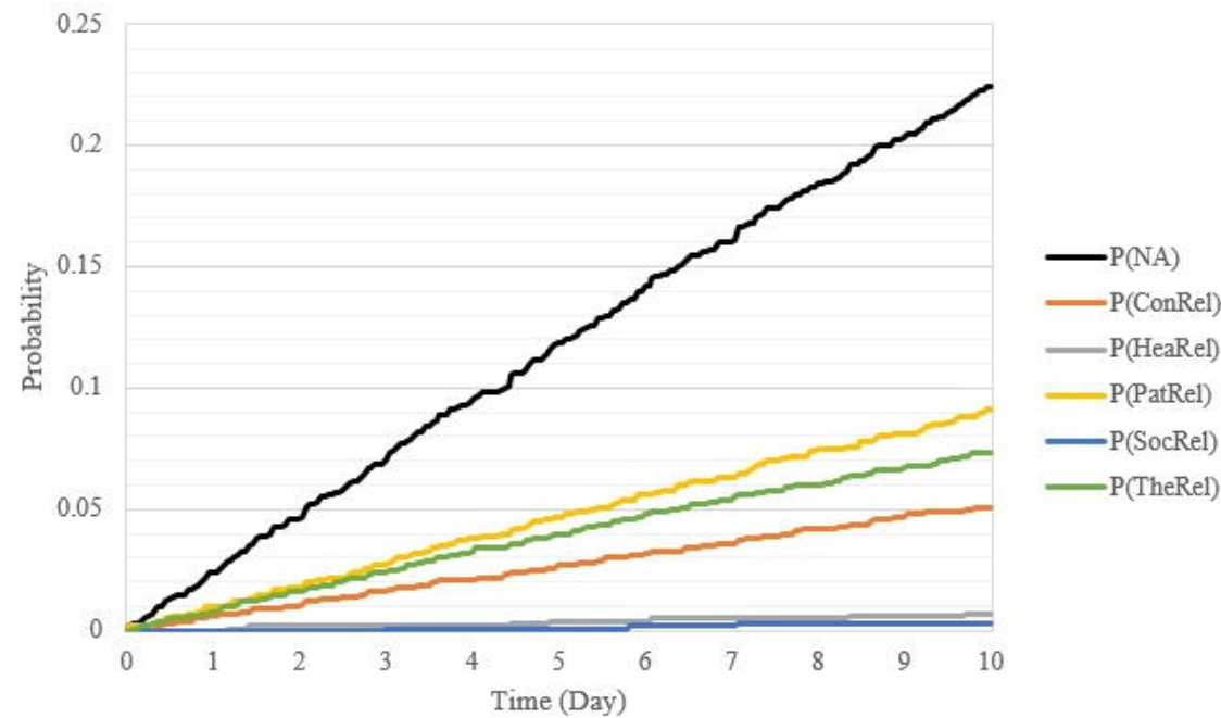
P(NA) and P(NAFs)
