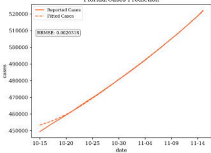
Florida:Cases Prediction
