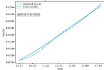
Maryland:Deaths Prediction
