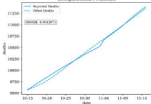
Georgia:Deaths Prediction
