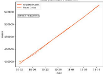
Georgia:Cases Prediction
