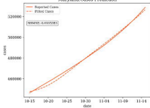
Maryland:Cases Prediction
