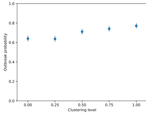
(d) Transmission probability = 0.55 ( \hat{R}_0 = 16.76 )
